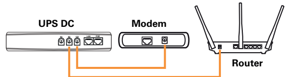
Modem y Router con distinto voltaje de alimentación
