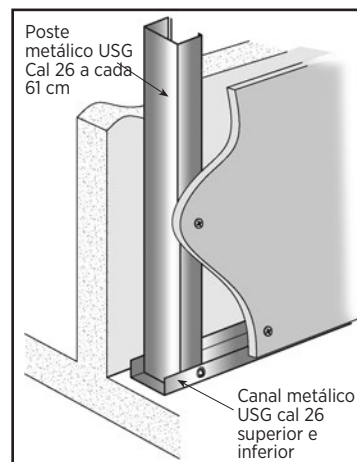
Lambrín a base de poste y canal
