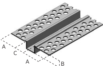
Junta de Control Recta
